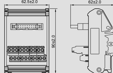
DM72-IDC-20-20-4Y-00Z(H)
