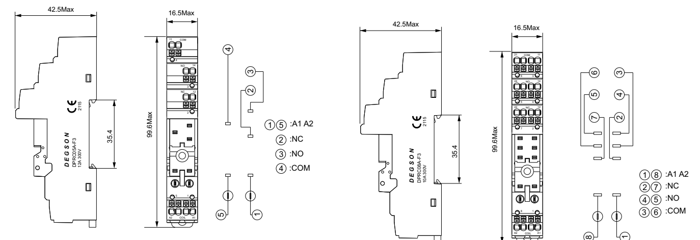
DPRC05A-F3
