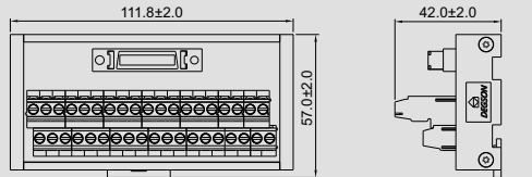
DM50-MDR-36-36-4Y-00Z(H)
