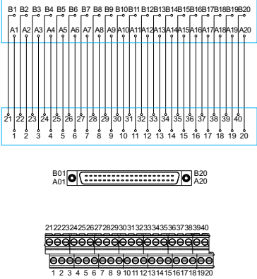
DM50-FCN-40-40-4Y-00Z(H)
