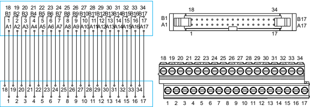
DM72-IDC-34-34-4Y-00Z(H) DM50-IDC-34-34-4Y-00Z(H)
