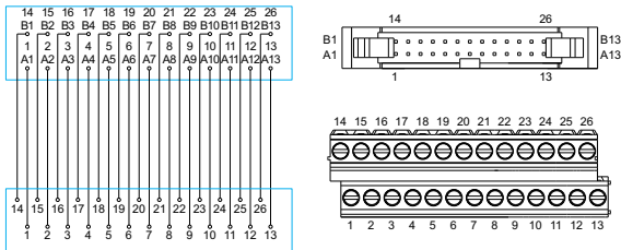
DM72-IDC-26-26-4Y-00Z(H) DM50-IDC-26-26-4Y-00Z(H)
