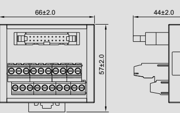
DM50-IDC-20-20-4Y-00Z(H)
