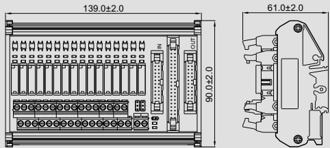
DM72-RMUS-16-PN-1-4M-00Z(H)
